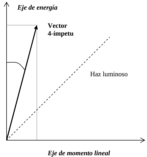
FIGURA 1. Arriba se ofrece una representación esquemática de un vector 4-ímpetu, en una gráfica bidimensional, donde el eje vertical es el de las energías y el horizontal el correspondiente al momento lineal. Obviamente, cuando la velocidad relativa se anula, el vector coincidiría con el eje de ordenadas: la energía propia coincide con la energía relativa.
